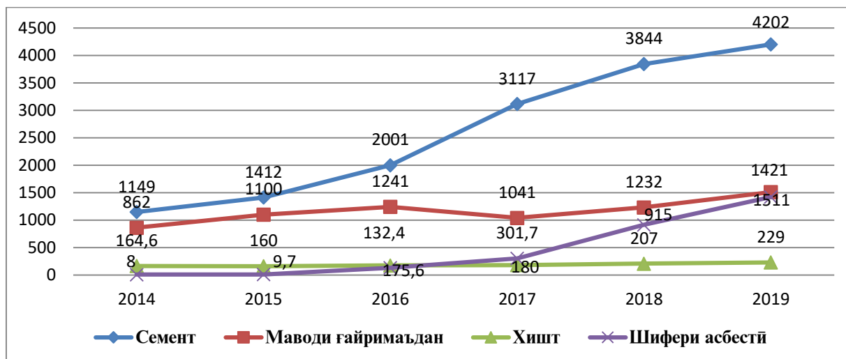
Расми 3. Истеҳсоли намудҳои асосии масолеҳи сохтмонӣ тӯли солҳои 2014-2019
